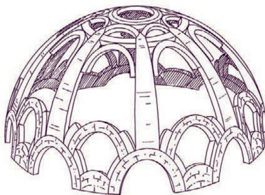
8. kép. A kupola szerkezete
